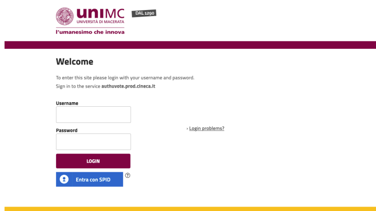
Figura 1: Autenticazione.
